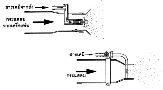
ภาพที่ 5 การเกิดของละอองสารจากหัวฉีดชนิดใช้แรงลม ภาพบนละอองเกิดจากกระแสลม และใบพัดตีของเหลวให้แตกกระจาย ภาพล่างละอองเกิดจากกระแสลมตีของเหลวให้แตกกระจาย
