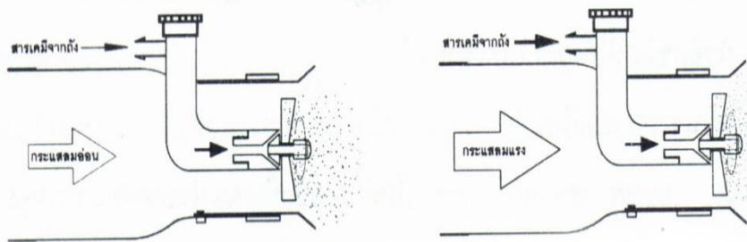
ภาพที่ 5 การเกิดของละอองสารจากหัวฉีดชนิดใช้แรงลม ภาพบนละอองเกิดจากกระแสลม และใบพัดตีของเหลวให้แตกกระจาย ภาพล่างละอองเกิดจากกระแสลมตีของเหลวให้แตกกระจาย
