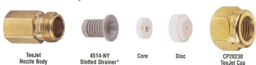
ภาพที่ 1 ชิ้นส่วนต่าง ๆ ของหัวฉีดชนิดใช้แรงดันของเหลว
